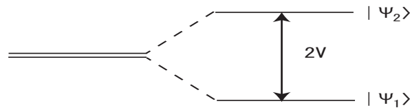
図 1: 相互作用が斥力的な場合の縮退した 2 準位系の相互作用によるエネルギー分岐
