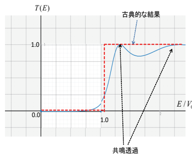
図 10: 矩形型ポテンシャルにおける透過率のエネルギー依存性
